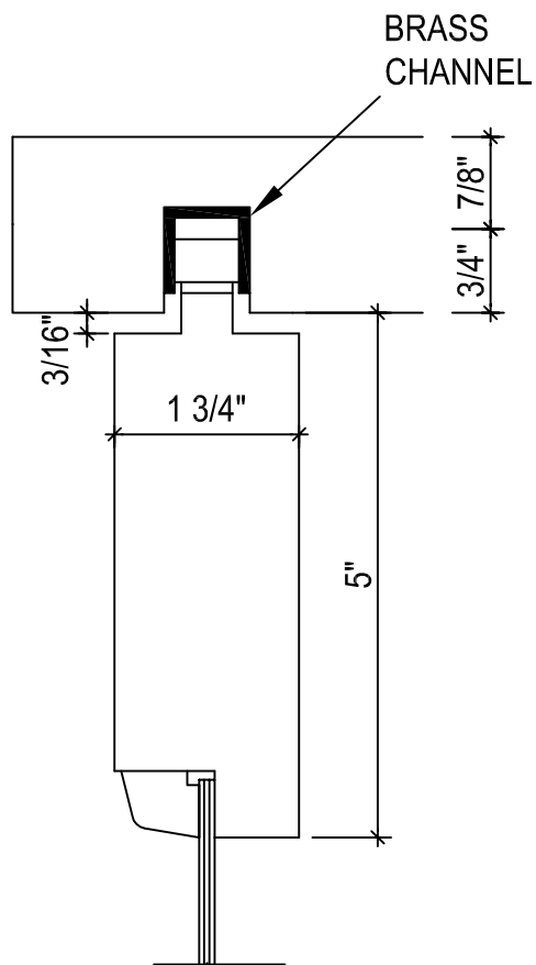
SLIDING DOOR TOP RAIL
